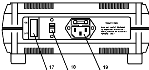
Рисунок 4. Задняя панель.
